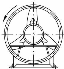
Виконання 2 (ліве обертання)
