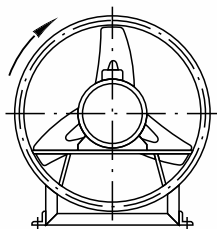
Виконання 1 (праве обертання)
