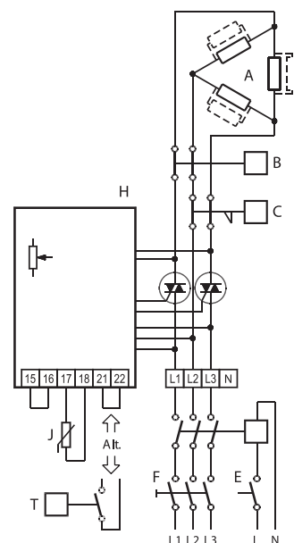
CBM-3 400В 3~
