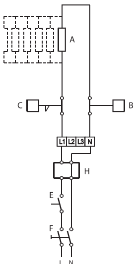
CB-1 230В~
