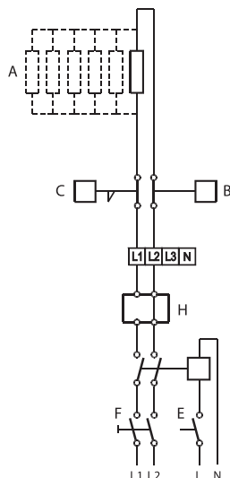
CB-2 400В 2~
