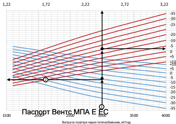
Витрата повітря через теплообмінник, м³/год
